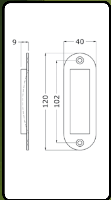
schuifdeurkom 120 mm Art.nr. 4560
